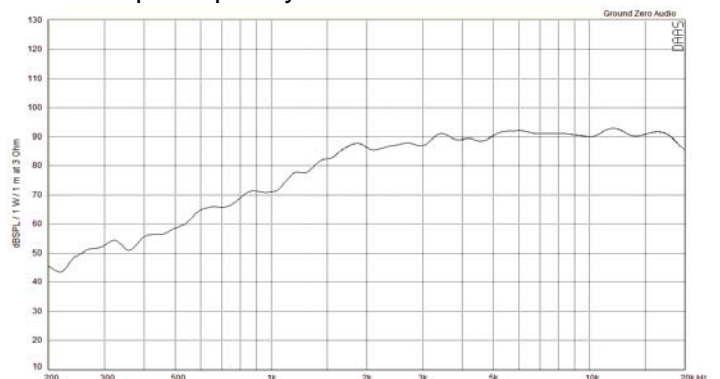
Frequenzgang / Frequency Response / Réponse en fréquence Verloop Frequency
