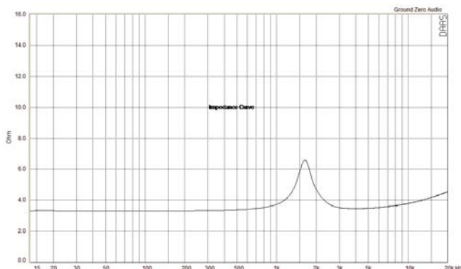
Impedanzverlauf / Impedance Curve / Frequency Verloop
